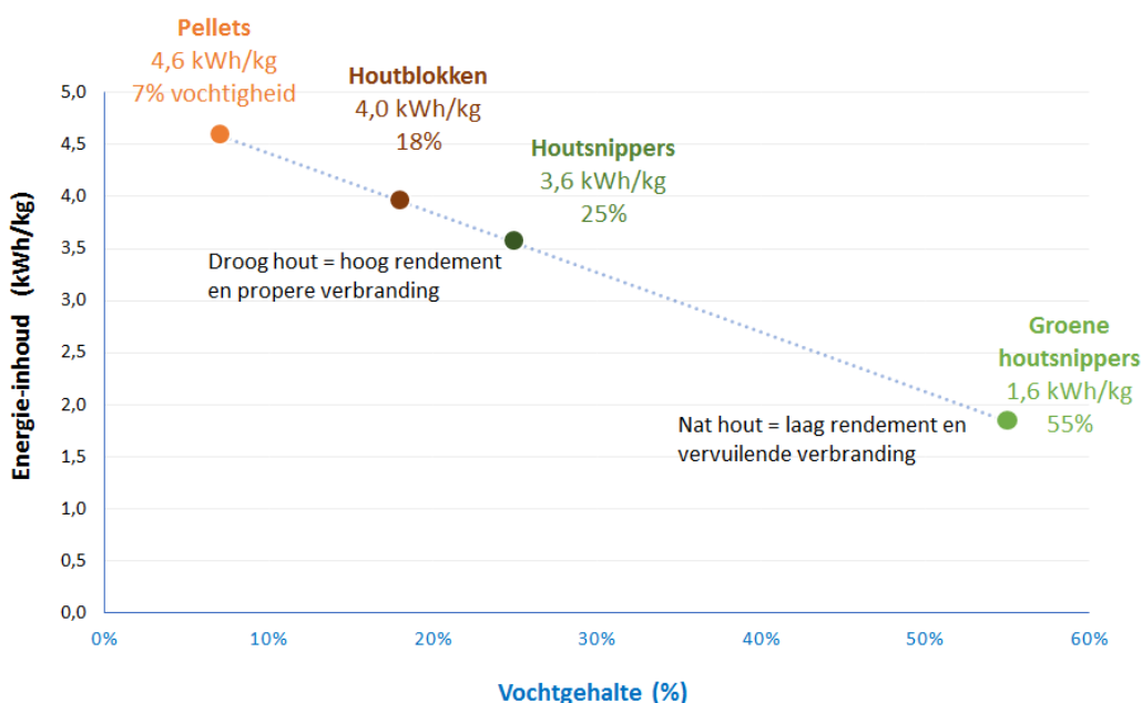
Afbeelding 3.3: Energie-inhoud van houtachtige brandstoffen in relatie tot het vochtgehalte (bron: www.ode.be)
