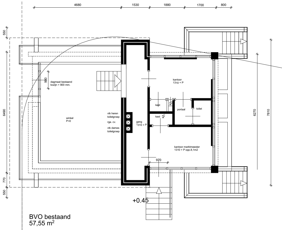
BEGANE GROND
