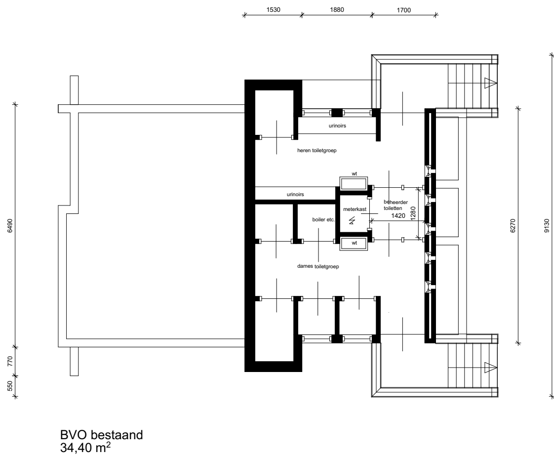
SOUTERRAIN
